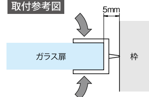
取付参考図
