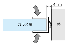
取付参考図
